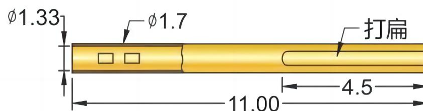
R1051 焊接片
